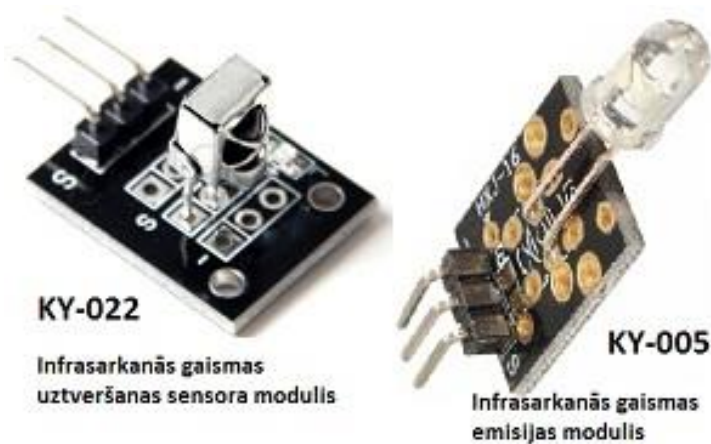
2. att. Infrasarkanās gaismas sensori
